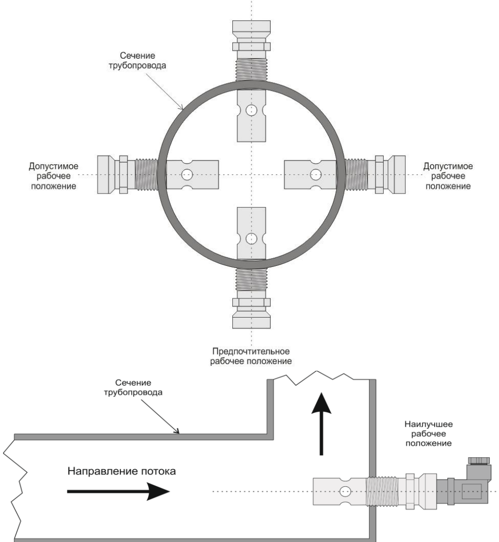
«Допустимые положения датчиков ДЭТ9 на трубопроводе»
