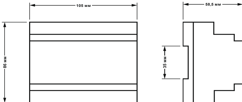
«Габаритные и установочные размеры Блока СЛ23»
